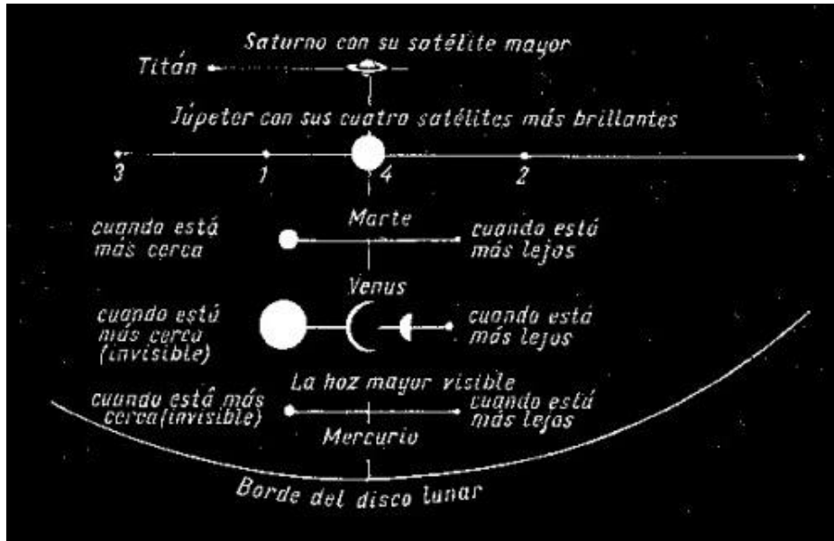
Figura 128. Si este dibujo se mira desde 25 cm de distancia los discos de los planetas que figuran en él se ven con las mismas dimensiones que cuando se observan estos planetas con un telescopio de 100 aumentos.
