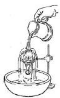
Figura 87. El agua del frasco hierve cuando se le echa agua fría
