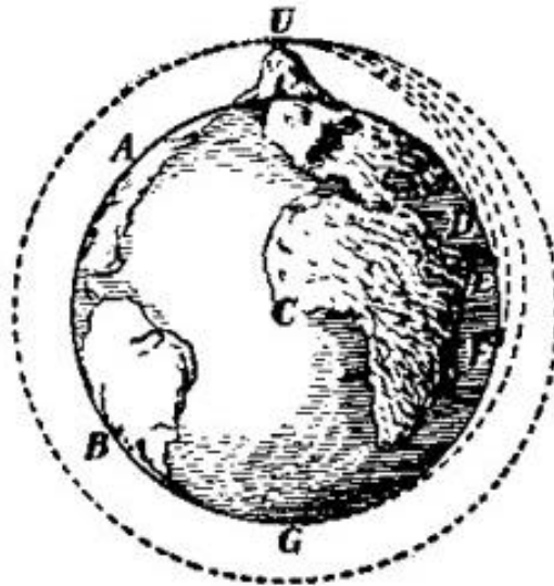
Fig. 50. Así deberían caer las piedras que se
